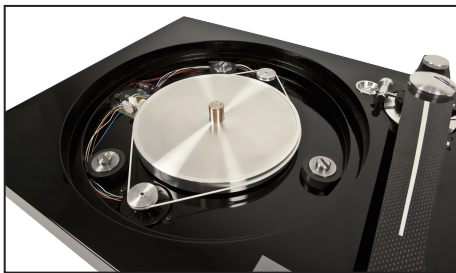
2台のモーターを内部に収納したベルトドライブ設計
